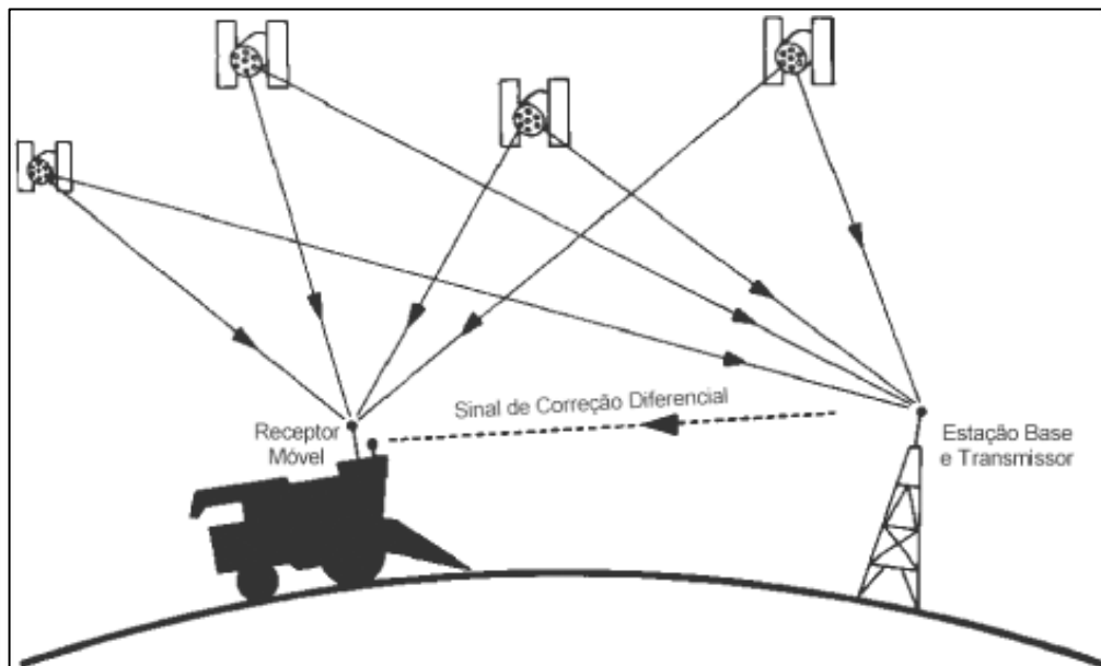
FIGURA 2 – Exemplo de utilização do sistema DGPS. Fonte: Scielo
