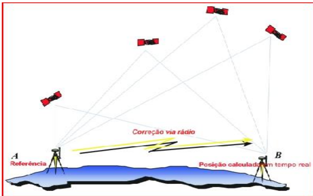
FIGURA 3 – Exemplo de utilização do sistema RTK. Fonte: MundoGEO
